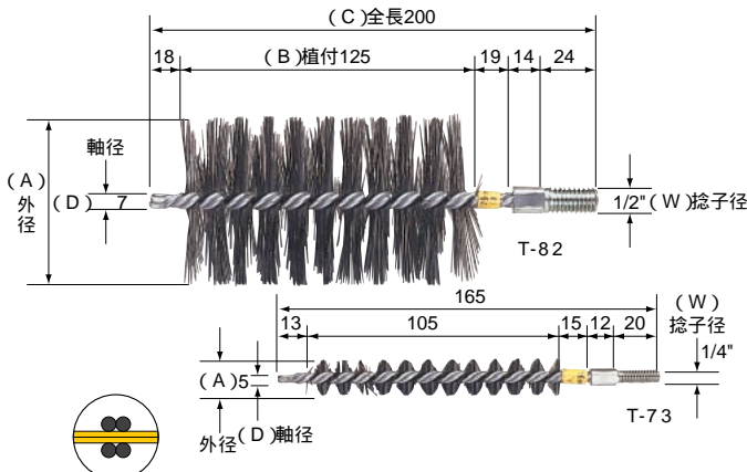
ダブルシングルスパイラル巻 1/4・1/2捻子用つなぎ柄は31ページに記載しています。
