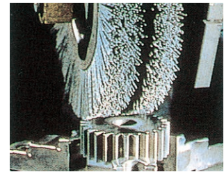
DISC-CENTER:ギヤーのバリ取り
