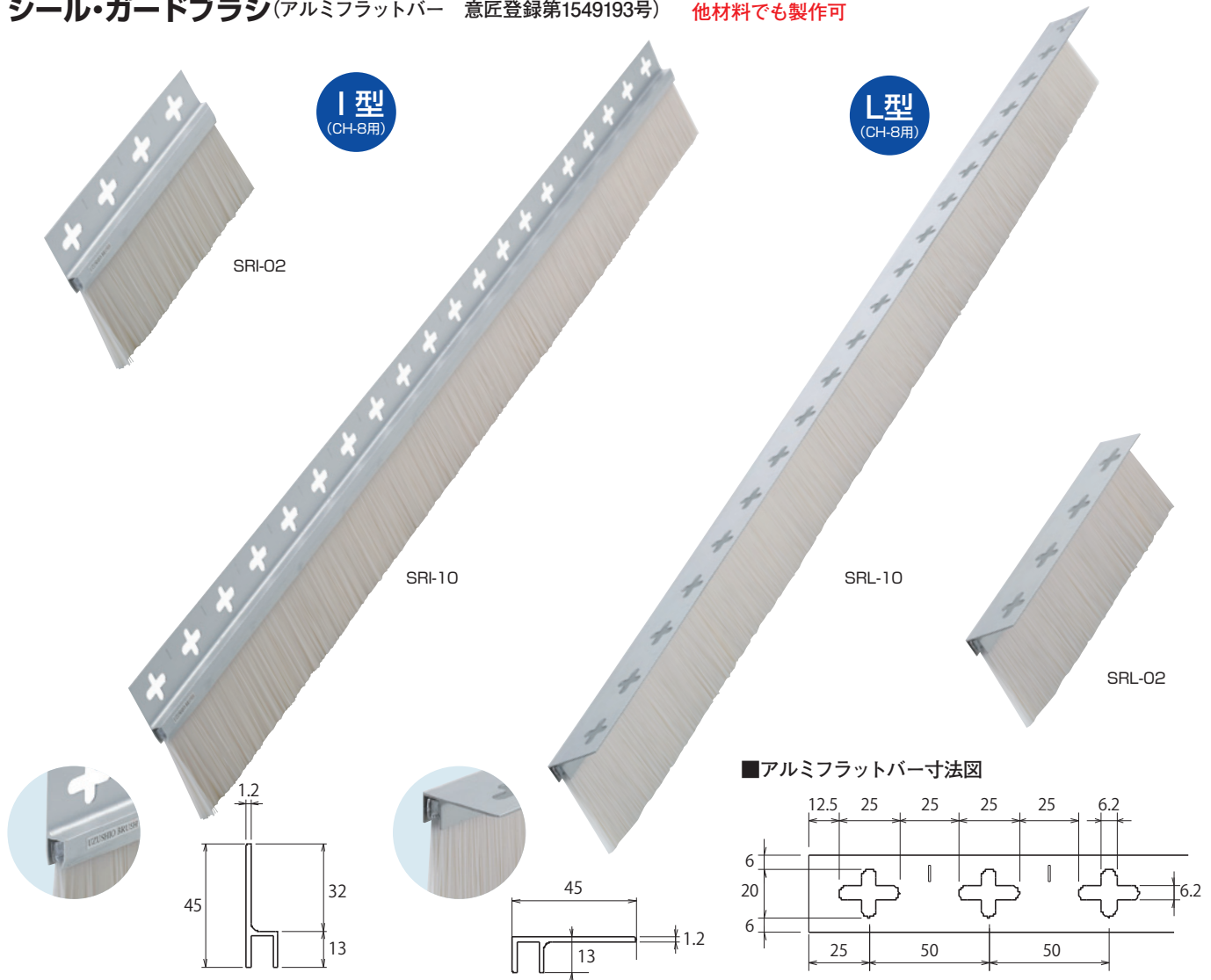
I型 シール・ガードブラシ(イオンスレッド・ハード植)
