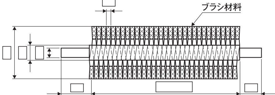
シャフト段付チャンネル密接左巻ロールブラシ
