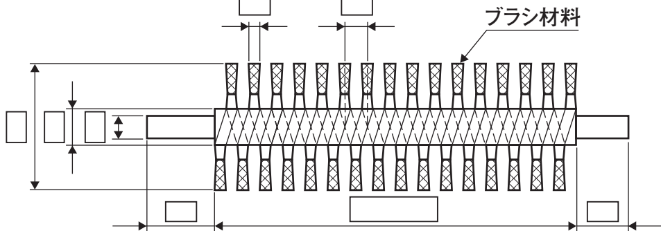
シャフト段付チャンネル間隔左巻ロールブラシ
