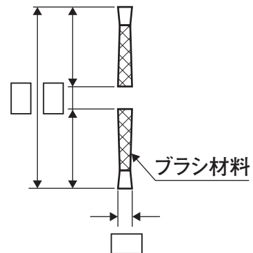
チャンネル内巻リングブラシ
