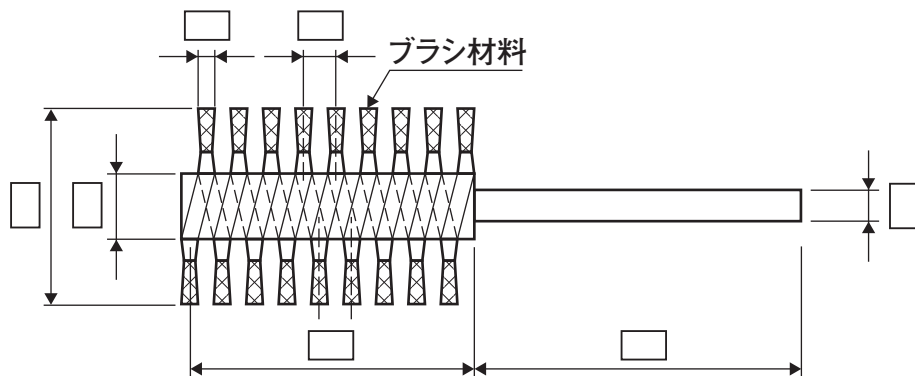
段付片軸付チャンネル間隔左巻ロールブラシ
