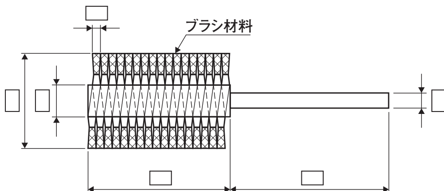
段付片軸付チャンネル密接 左巻ロールブラシ
