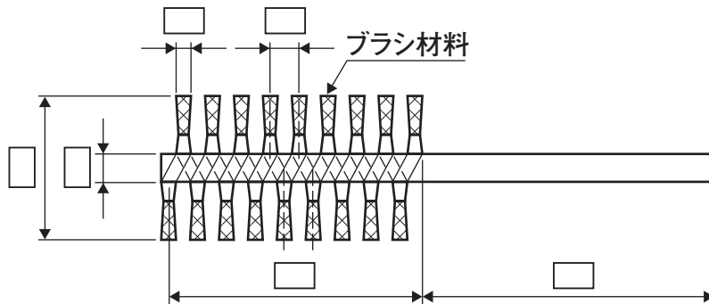
片軸付チャンネル間隔左巻ロールブラシ
