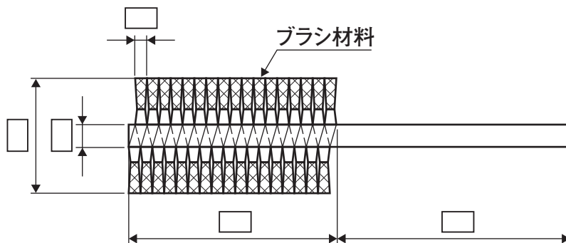
片軸付チャンネル密接左巻ロールブラシ
