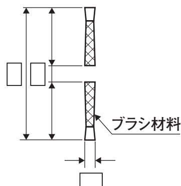
チャンネル内巻リングブラシ
