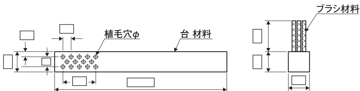
台回転ブラシ
