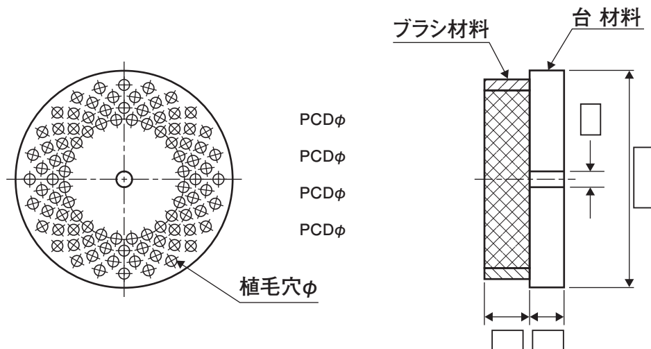
台ポリッシャーブラシ
