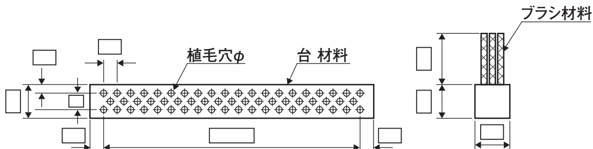
台長方形ブラシ
