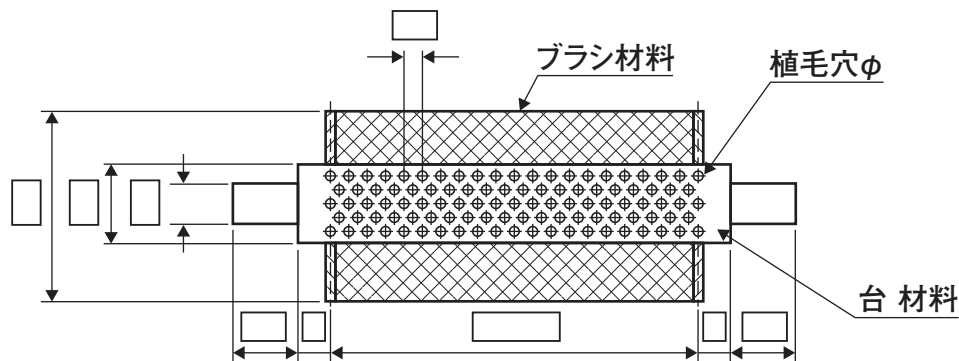
シャフト付 台ロールブラシ チドリ植
