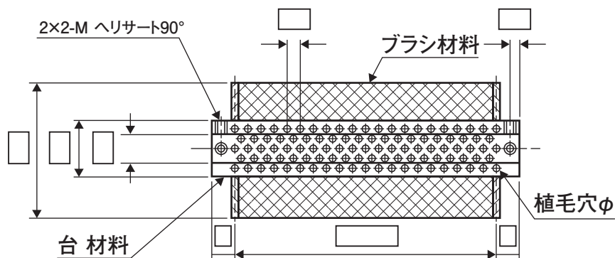
シャフトなし 台ロールブラシ チドリ植
