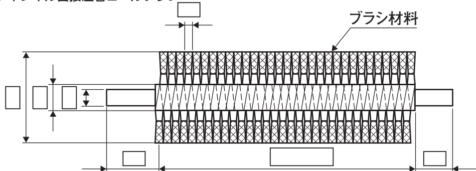
シャフト段付チャンネル密接左巻ロールブラシ
