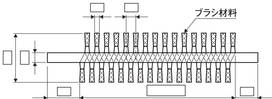
シャフト付チャンネル間隔左巻ロールブラシ
