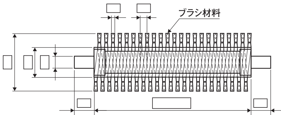
シャフト・ドラム付チャンネル間隔左巻ロールブラシ
